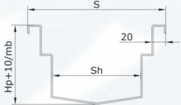
Przekrój kanału z dnem łamany
